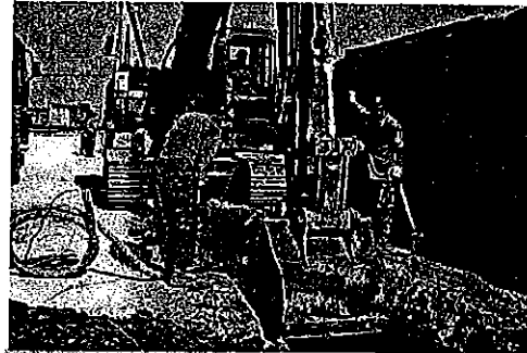
側溝工事の様子
