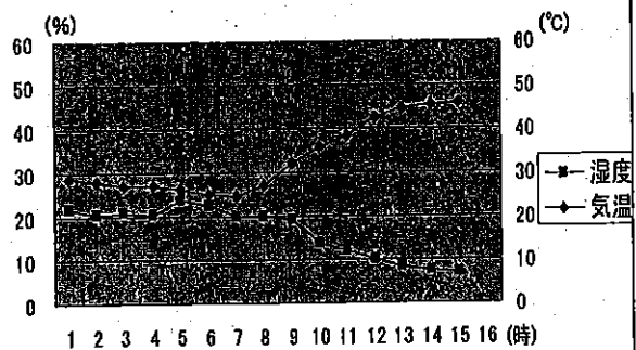
気温・湿度推移(サマータイム)
